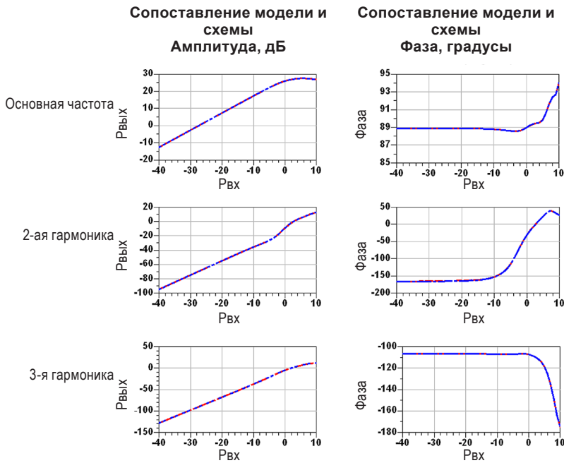
Рис. 2. Представленные здесь X-параметры сопоставляются с результатами анализа реальной схемы. Очевидно, что X-параметры точно соответствуют реальной схеме.
