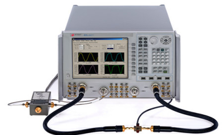
Рис. 3. ПО нелинейного векторного анализа, предназначенное для использования в анализаторе цепей PNA-X компании Keysight, представляет новый промышленный стандарт анализа нелинейных ВЧ/СВЧ цепей в диапазоне от 10 МГц до 50 ГГц. Это позволяет инженерам измерять X-параметры в полном объеме.
