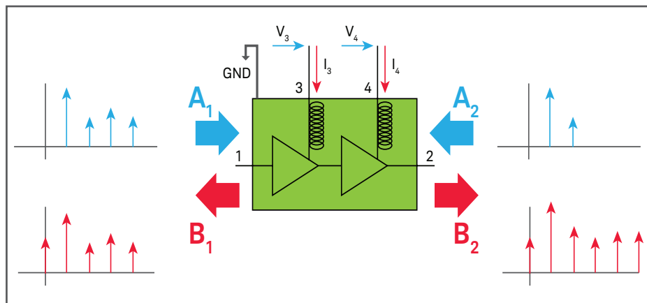
Рис. 1. В этом примере созданная в частотной области модель многокаскадного усилителя на основе X-параметров отображает связь прямых (A) и отраженных волн (B). Так как все значения амплитуды и фазы прямой и отраженной волн на всех гармониках точно соответствуют значениям во временной области, то в результате можно зарегистрировать полные нелинейные входные и выходные характеристики устройства.
