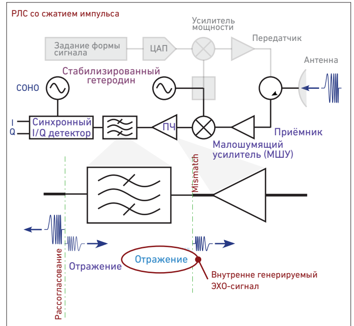
Рисунок 1. Отражения из-за рассогласования могут быть причиной появления паразитных эхо-сигналов
