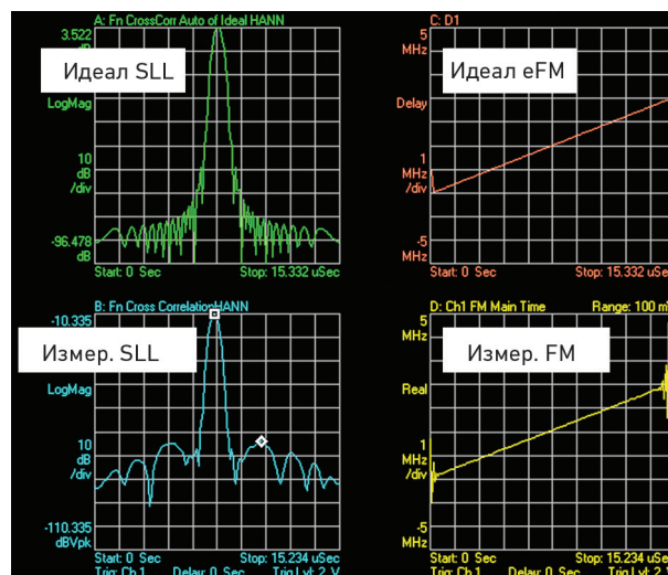
Рисунок 4. Измерение уровня боковых лепестков SLL
