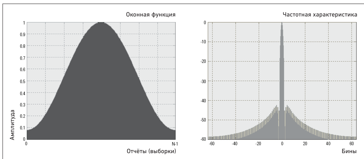
Рисунок 2. Оконная функция Хэмминга и соответствующая ей частотная характеристика
