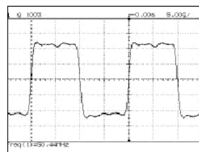
50МГц прямоугольный сигнал на экране 500МГц осциллографа
