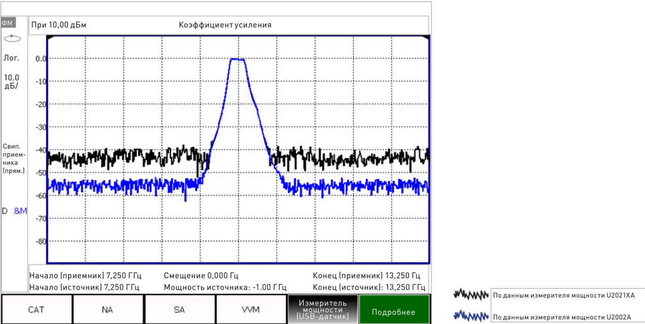
Пример, показывающий типичный динамический диапазон измерения FOPS
