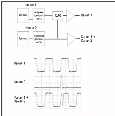
Рисунок 2 - Суммирование каналов
