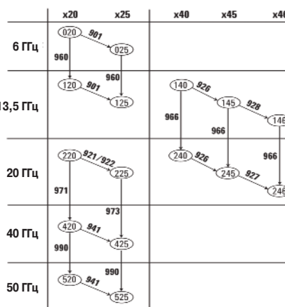
Примеры путей модернизации анализаторов цепей серии PNA-L
