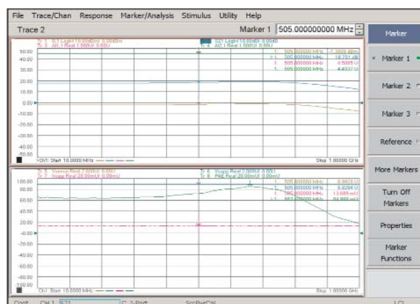
Рисунок 33 - Результаты измерения КПД добавленной мощности
