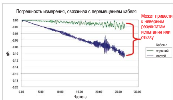
Рисунок 42 - Влияние перемещения кабеля на точность измерения после калибровки
