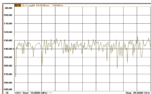
Рисунок 50 - Зависимость уровня собственных шумов анализатора цепей PNA-X с непосредственным подключением к приёмнику от частоты (тип. значения)
