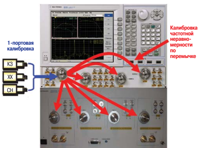
Рисунок 44 - Процесс проведения калибровки QSOLT
