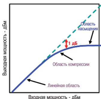
Рисунок 23 - Принцип измерения компрессии усиления
