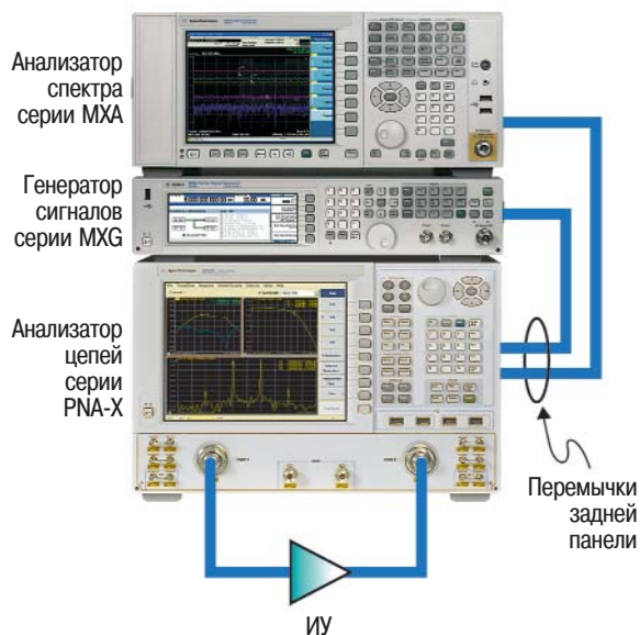
Рисунок 34 - Расширение набора измерений при одном подключении к ИУ за счёт добавления внешних векторных генераторов сигналов и анализаторов
