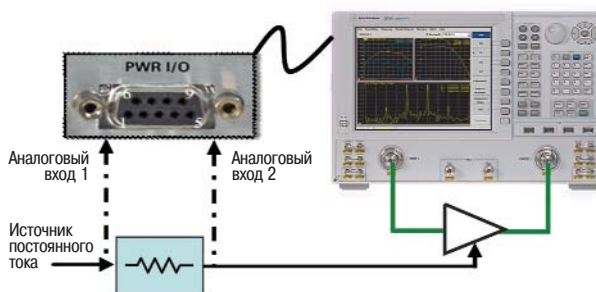
Рисунок 31 - Конфигурация установки для измерения КПД добавленной мощности
