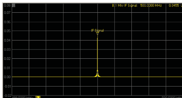
Рисунок 15 - Результаты широкополосного цикла свипирования
