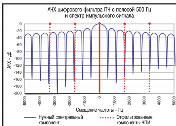
Рисунок 1 - Спектральное обнуление
