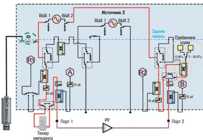
Рисунок 21 - Техническое решение для измерения коэффициента шума на базе PNA-X (до 26,5 ГГц)
