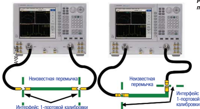
Рисунок 41 - Калибровка по неизвестной перемычке
