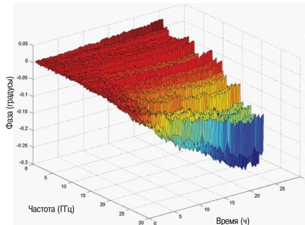
Рисунок 48 - PNA-X по истечении 24 часов: зависимость дрейфа фазы S_{11} от времени 1,2
