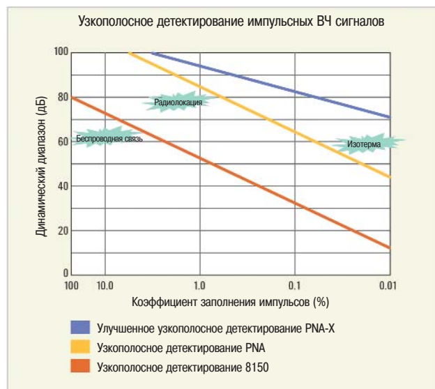
Рисунок 3 - Сравнение характеристик узкополосного детектирования
