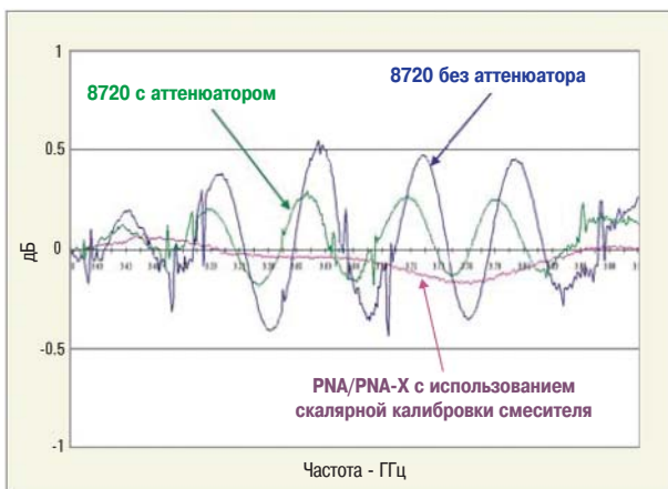
Рисунок 7 - Сравнение результатов измерения потерь преобразования
