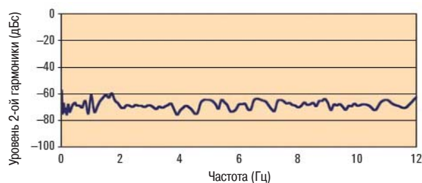
Зависимость уровня гармоник источника анализатора цепей PNA-X от частоты (тип. значения)
