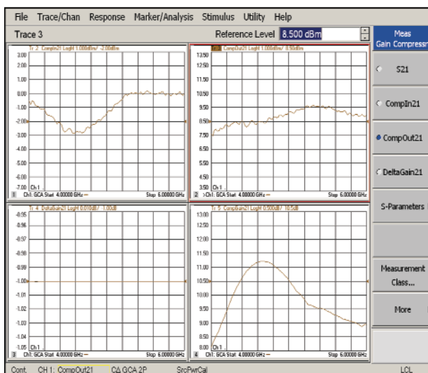
Рисунок 25 - Результаты измерения компрессии коэффициента усиления в режимах свипирования
