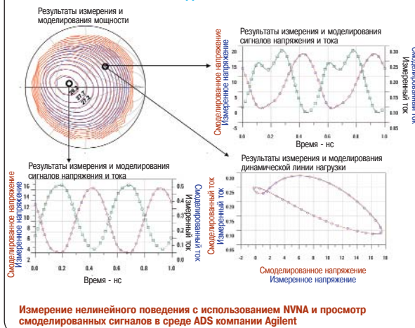
Рисунок 37 - Сравнение результатов, полученных при фактических измерениях, с результатами, полученными при моделировании в среде ADS с использованием X-параметров, показывает удивительную взаимосвязь
