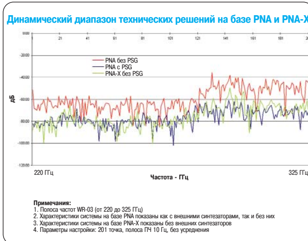
Рисунок 38 - PNA-X обеспечивает превосходный динамический диапазон до 325 ГГц, не требуя использования внешних ВЧ генераторов сигналов и источников сигнала гетеродина
