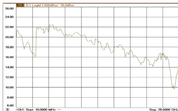
Рисунок 49 - Зависимость выходной мощности источника полностью сконфигурированного анализатора цепей PNA-X от частоты (тип. значения)
