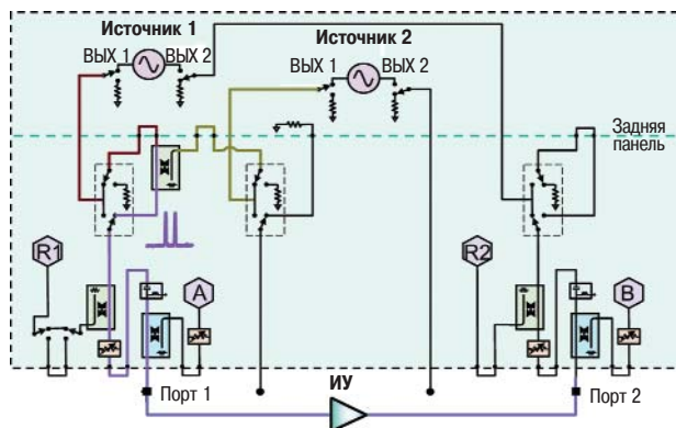
Рисунок 27 - Структурная схема PNA-X при измерении интермодуляционных искажений
