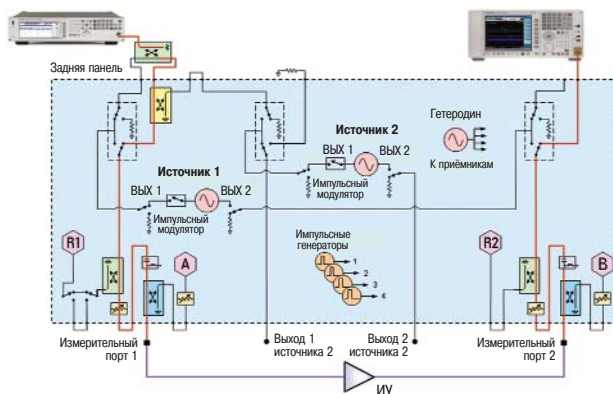
Рисунок 35 - Структурная схема, показывающая подсоединение генератора сигналов и анализатора спектра для расширения набора измерений ВЧ сигналов
