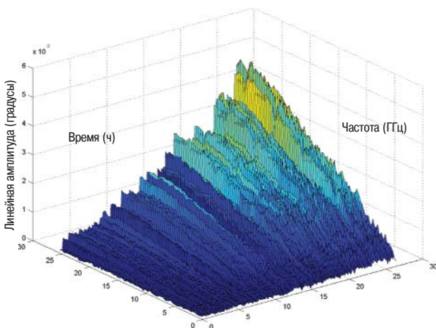
Рисунок 47 - PNA-X по истечении 24 часов: зависимость дрейфа амплитуды S_{11} от времени 1,2
