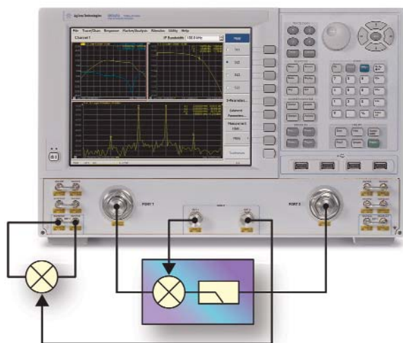
Рисунок 13 - Калибровка преобразователя частоты со встроенным гетеродином
