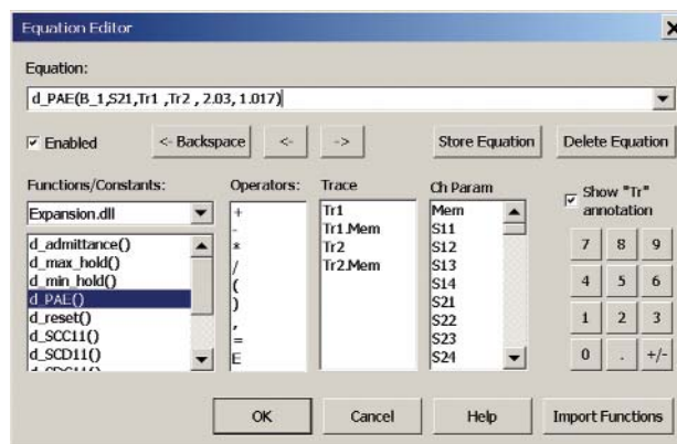
Рисунок 29 - Вычисление КПД добавленной мощности с использованием редактора формул (Equation Editor)
