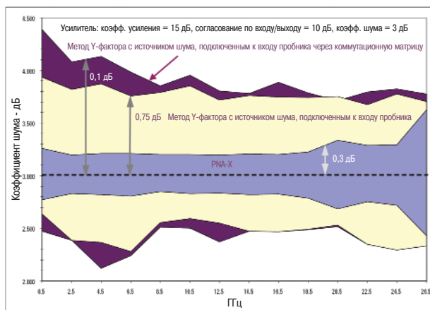
Рисунок 22 - Сравнение погрешностей измерения коэффициента шума
