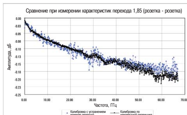
Рисунок 43 - Сравнение точности методов калибровки по неизвестной перемычке и калибровки с устранением влияния перехода
