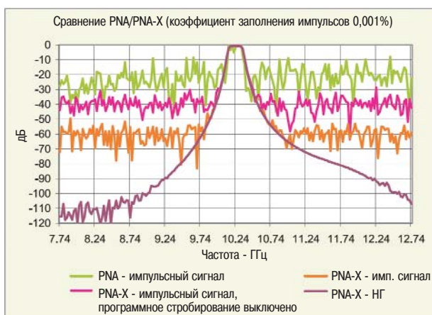
Рисунок 6 - Сравнение PNA-X и PNA при измерении параметров цепей в импульсном режиме
