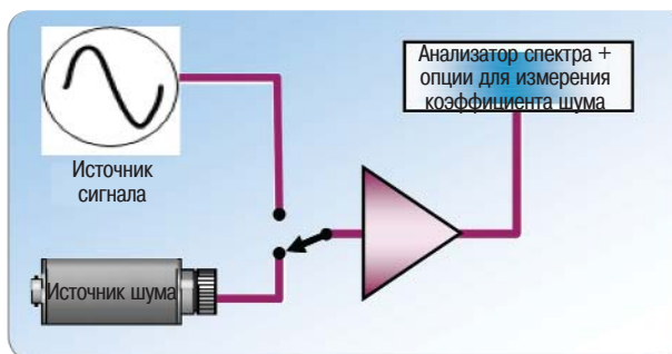
Рисунок 20 - Автоматизированная испытательная система
