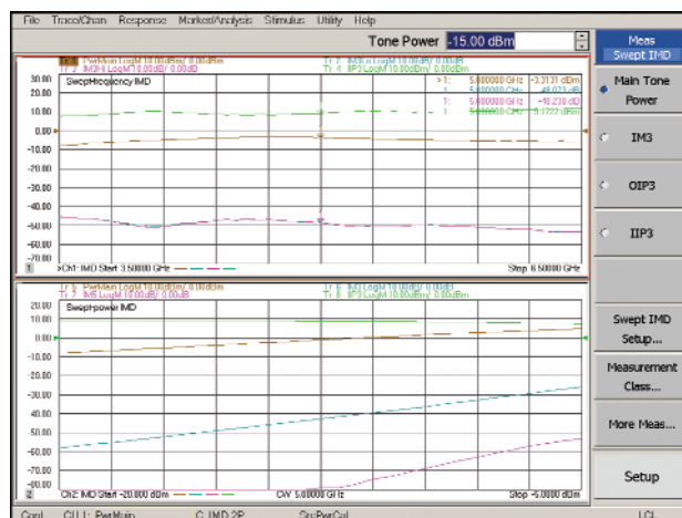
Рисунок 28А - Результаты измерения интермодуляционных искажений в режимах свипирования по частоте и свипирования по мощности с использованием анализатора цепей PNA-X
