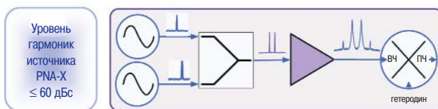
Рисунок 26 - Измерение интермодуляционных искажений
