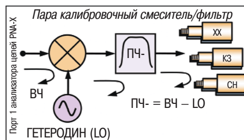
Рисунок 10 - Характеристики калибровочного смесителя определяются посредством выполнения трёх измерений параметров отражения с использованием в качестве нагрузки мер холостого хода (XX), короткозамкнутой нагрузки (КЗ) и согласованной нагрузки (СН).
