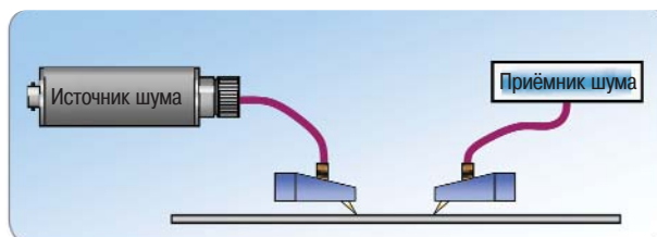
Рисунок 19 - Зондовое измерение компонентов на пластинах
