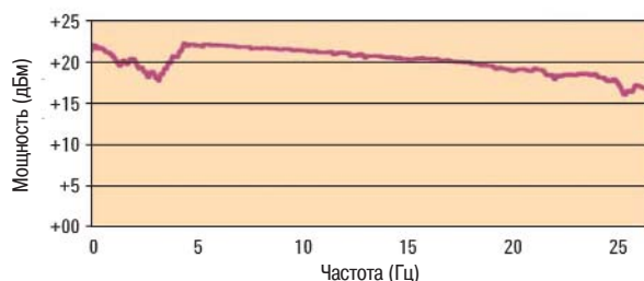
Зависимость выходной мощности анализатора цепей PNA-X от частоты (тип. значения)
