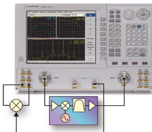
Рисунок 14 - Измерение характеристик преобразователя частоты со встроенным гетеродином
