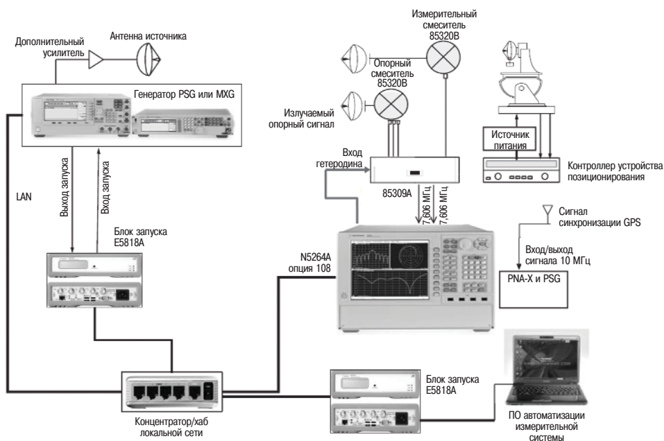
Рисунок 40 - Типовая конфигурация для измерения параметров антенн в дальней зоне с использованием измерительного приёмника на базе анализатора цепей PNA-X компании Agilent
