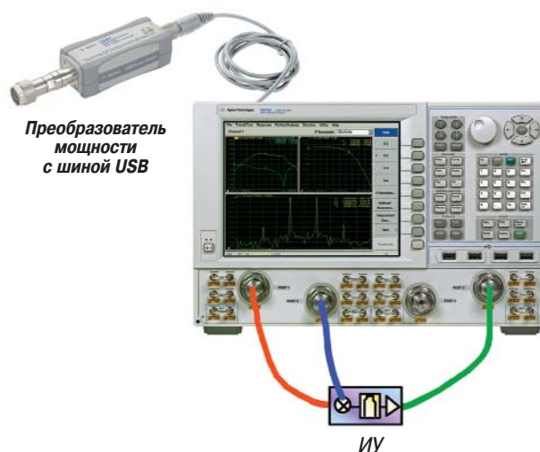
Рисунок 8 - Конфигурация измерительной установки для скалярной калибровки смесителя
