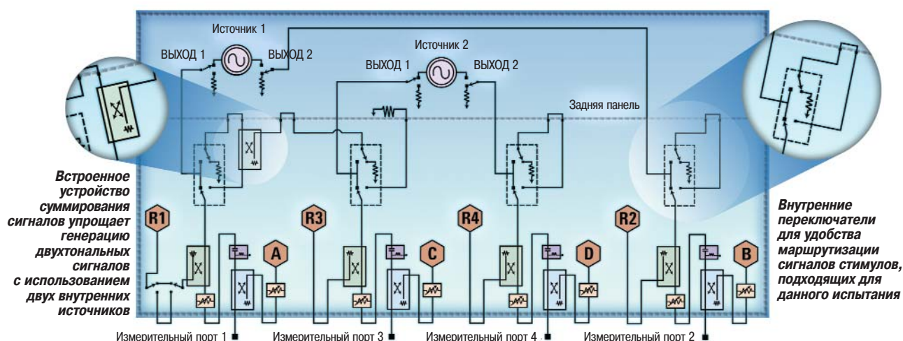
Структурная схема анализатора цепей серии PNA-X (показана с опциями 400, 419 и 423)
