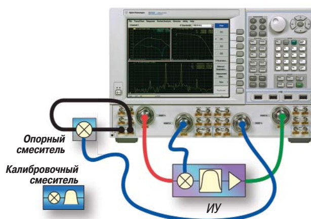
Рисунок 9 - Конфигурация измерительной установки для векторной калибровки смесителя
