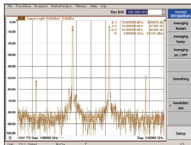
Рисунок 28В - Режим отображения спектра интермодуляционных искажений анализатора цепей PNA-X, формирующий отображение сигналов, как в анализаторе спектра
