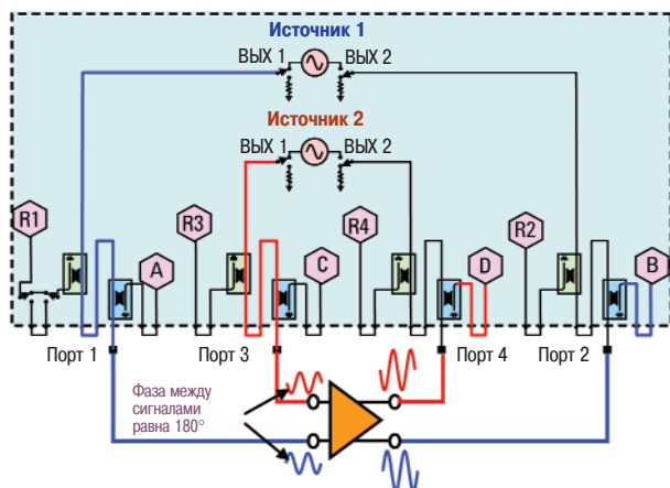
Рисунок 29 - Измерения с использованием истинных дифференциальных сигналов
