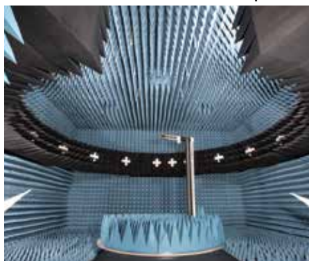
Испытательные системы AMS-8700 на базе безэховой камеры
