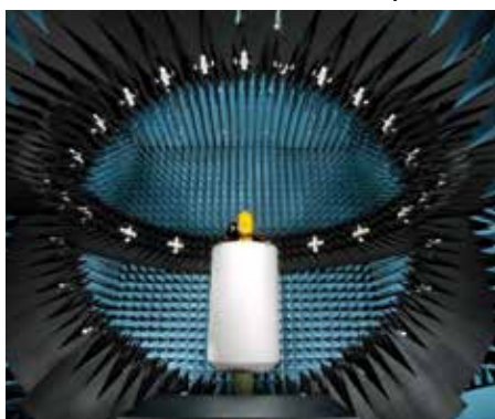
Испытательные системы AMS-8900 на базе безэховой камеры
