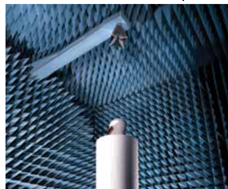
Испытательные системы AMS-8800 на базе безэховой камеры
