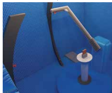
Испытательные системы для антенных измерений 5G / СВЧ
