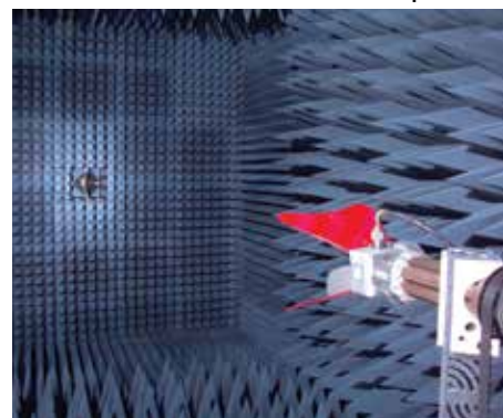
Испытательные системы AMS-8500 на базе безэховой камеры
