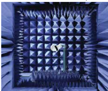
Испытательные системы AMS-8600 на базе безэховой камеры
