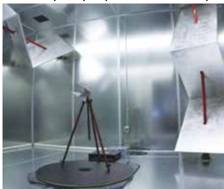
Испытательные системы AMS-7200 на базе реверберационной камеры
