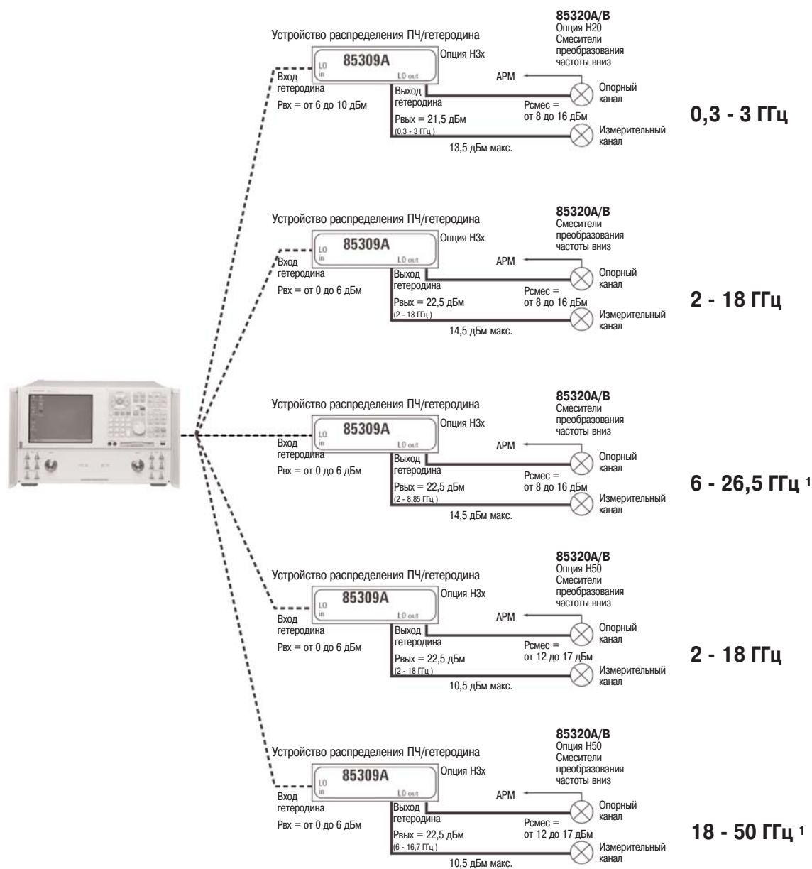
Рисунок 28 - Конфигурации устройства 85309A, оснащенного опцией H30, H31 или H32 с внешними смесителями
