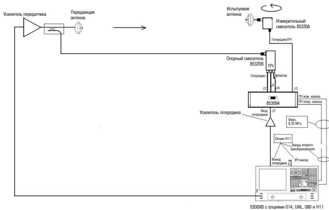
Рисунок 4 - Конфигурация для антенных измерений в поле дальней зоны с использованием внутренних источников серии PNA с опцией H11
