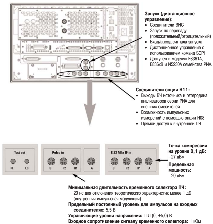
Рисунок 13 - Соединители задней панели
