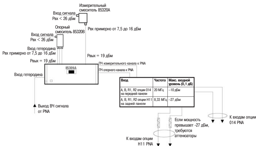
Рисунок 14 - Диаграмма соединений и требования к входным уровням для опций H11 и 014 серии PNA
