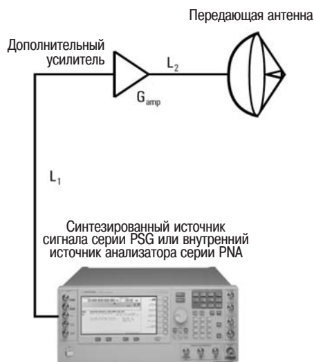
Рисунок 8 - Конфигурация передающей части
