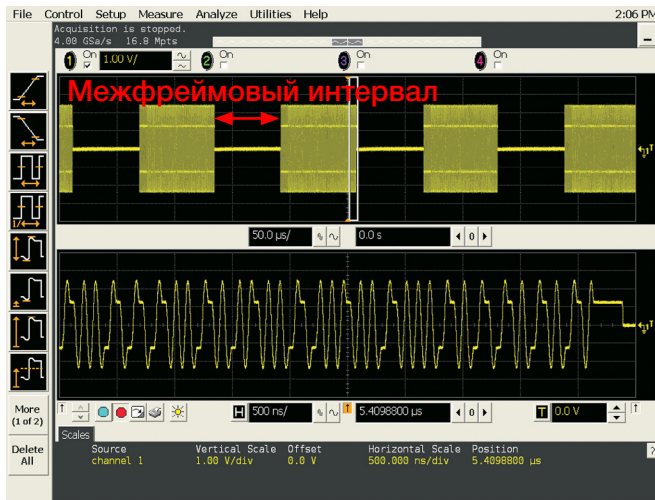
Рис.6. Случайная последовательность пакетов данных с Манчестерской кодировкой. В нижней части экрана показан увеличенный фрагмент сигнала, соответствующий белому прямоугольнику в верхней части экрана.
