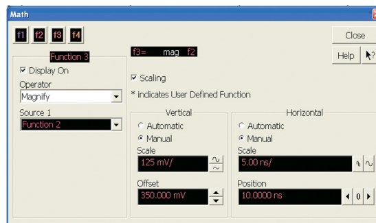
Рис. 14b. Функция 3 затем используется для усиления отфильтрованного с использованием функции 2 сигнала. Форма сигнала в точке А нормализуется путем деления на значение пикового напряжения в точке А.
