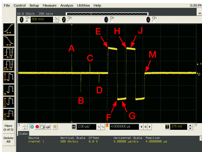
Рис. 13. Один период сигнала контрольного режима 1 с помеченными контрольными точками от A до M.
