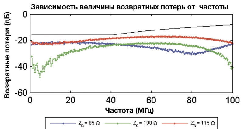
Рис. 17. График зависимости величины возвратных потерь устройства стандарта 1000BASE-T от частоты
