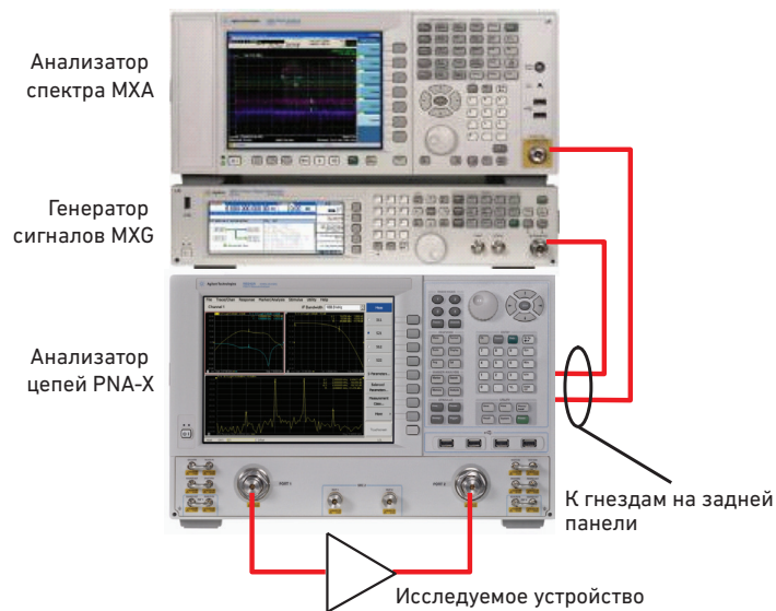
Рис. 2. Коммутаторы подают сигнал с генератора MXG на вход ИУ, а с выхода ИУ — на анализатор спектра MXA. Внешний направленный ответвитель подает сигнал PNA-X, обеспечивая связь через внутренний сумматор для двух встроенных источников сигнала — такая конфигурация используется для измерения интермодуляционных искажений.
