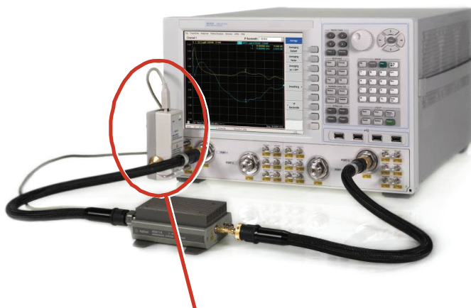
Уникальная методика калибровки коэффициента шума компании Keysight использует модуль ECal в качестве устройства согласования импеданса для устранения влияния рассогласования с источником
