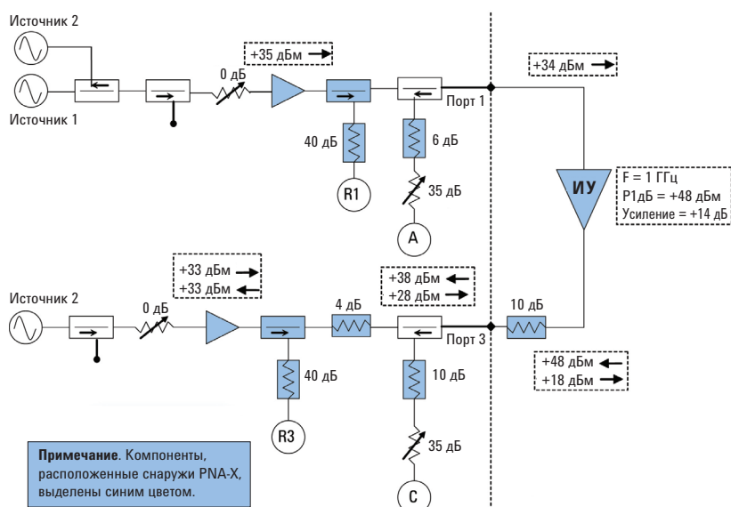
Рис. 2. Структурная схема системы тестирования усилителя с максимальной выходной мощностью +48 дБм.
