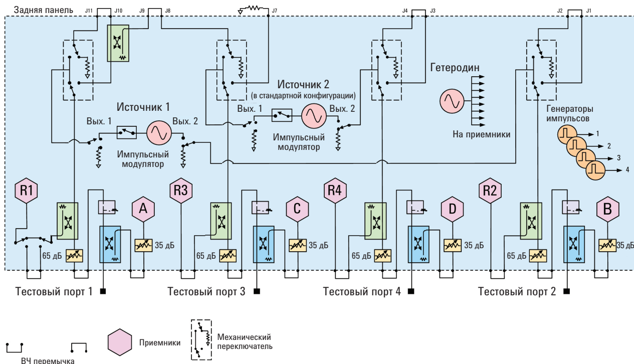
Рис. 1. Структурная схема PNA-X N5242A с опцией 423 для ВЧ испытаний.
