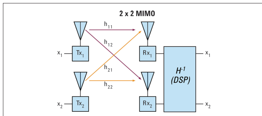
Рисунок 1в. Системы MIMO используют несколько антенн, пространственно-временное кодирование и алгоритмы оценки характеристик канала для создания нескольких пространственных каналов данных, передающих одинаковую информацию.
