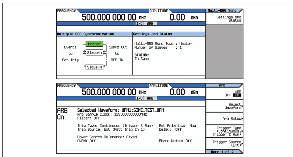
Рисунок 14. Генератор MXG с опцией 012 имеет функцию синхронизации нескольких генераторов модулирующих сигналов (MultiBBG Synchronization), которая используется для их временного выравнивания. Один прибор должен быть назначен ведущим, а другие ведомыми.
