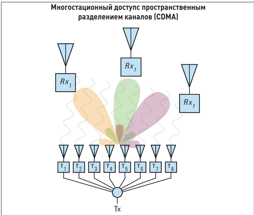
Рисунок 1d. Система SDMA использует формирование луча для передачи или приёма сигнала только от одного определённого передатчика или к одному определённому приёмнику.
