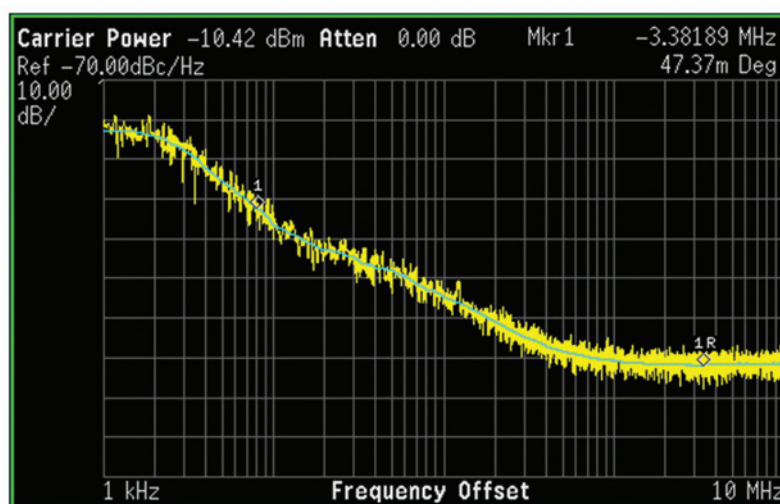
Рисунок 8. Полная фазовая ошибка, обусловленная фазовым шумом между источниками сигнала, может быть определена интегрированием некоррелированного фазового шума в пределах интегрирования, равных полосе сигналов, используемых в системе.
