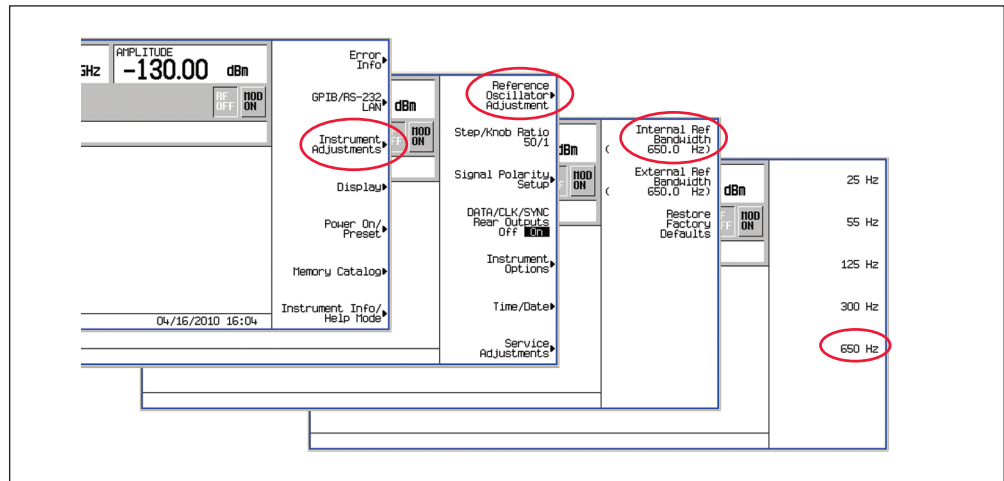
Рисунок 10. Для наилучшей фазовой стабильности между приборами, синхронизированными опорным сигналом, полосу опорного канала в генераторе PSG следует установить самой широкой с помощью опции UNX.
