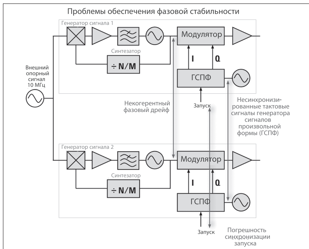
Рисунок 4. Синхронизация нескольких источников общим опорным сигналом с частотой 10 МГц обеспечивает лишь ограниченную фазовую стабильность между приборами.
