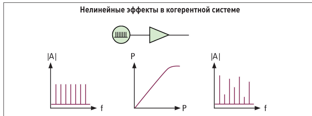
Рисунок 3. В когерентных системах продукты нелинейности могут комбинироваться непредсказуемым образом.
