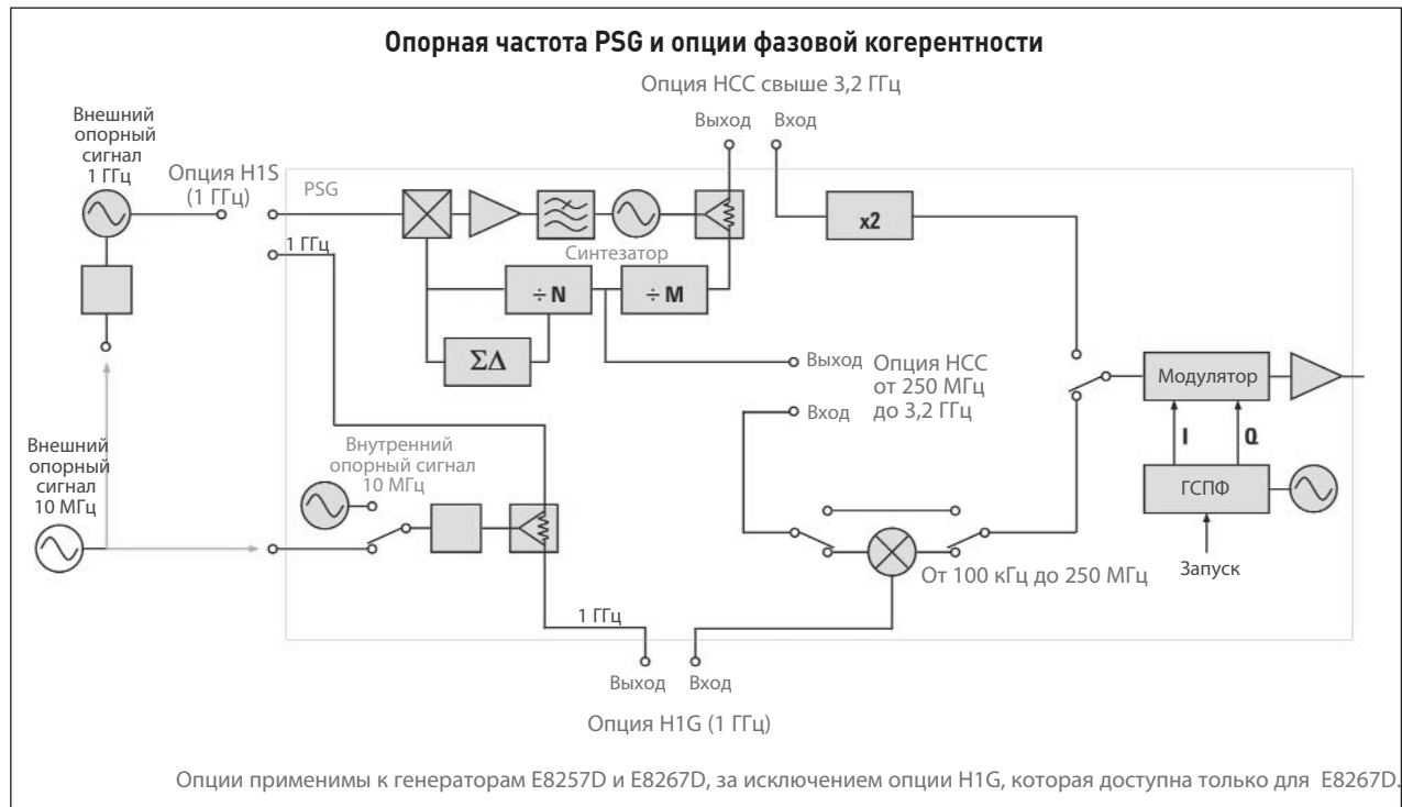
Рисунок 16. Опция HCC обеспечивает доступ к гетеродинам генераторов PSG с задней панели для трактов низкочастотной и высокочастотной полос. Опции H1S и H1G дают возможность использовать опорный сигнал 1 ГГц.
