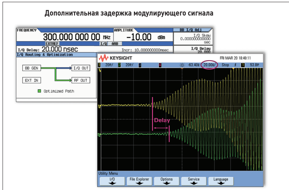
Рисунок 15. Генератор MSG с опцией 012 имеет функцию синхронизации нескольких генераторов модулирующих сигналов, используемую для выравнивания задержки между ними. Каждый прибор должен быть назначен ведущим или ведомым.
