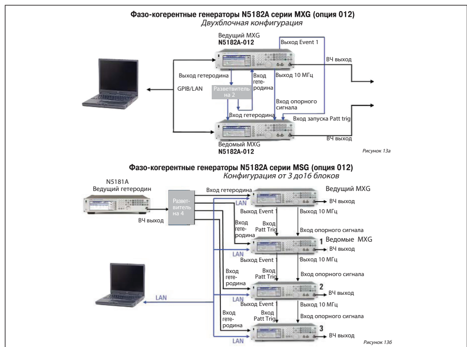
Рисунок 13. Эти когерентные конфигурации с несколькими генераторами MSG совместно используют общие гетеродины (опция 012).
