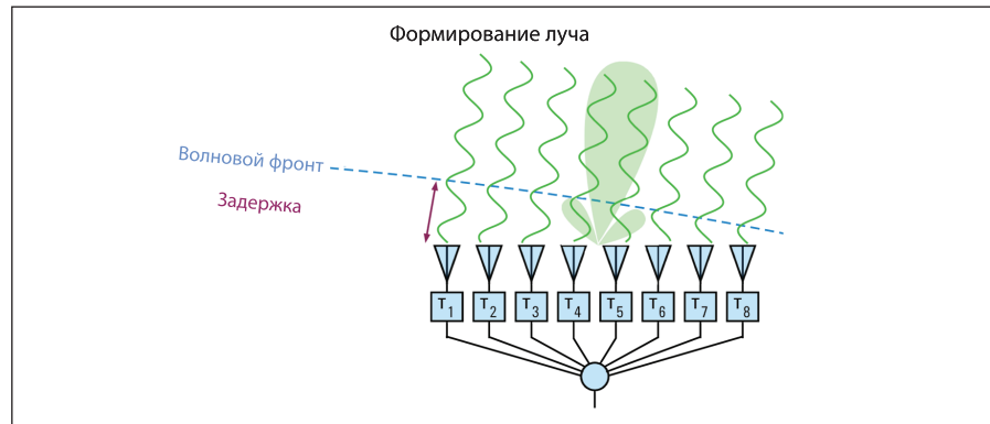
Рисунок 1с. Фазированная антенная решётка формирует луч путём настройки фазовых соотношений между когерентными антеннами таким образом, что сигналы объединяются конструктивно (суммируются) в нужном направлении и деструктивно (вычитаются) в других направлениях.
