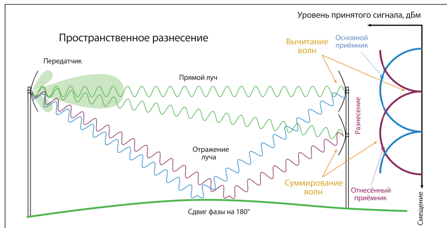
Рисунок 1а. Когерентный характер многолучевых сигналов заставляет их комбинироваться конструктивно (суммированием) или деструктивно (вычитанием). Хороший приём в условиях многолучевого распространения обеспечивается благодаря использованию пространственноразнесённых антенн.
