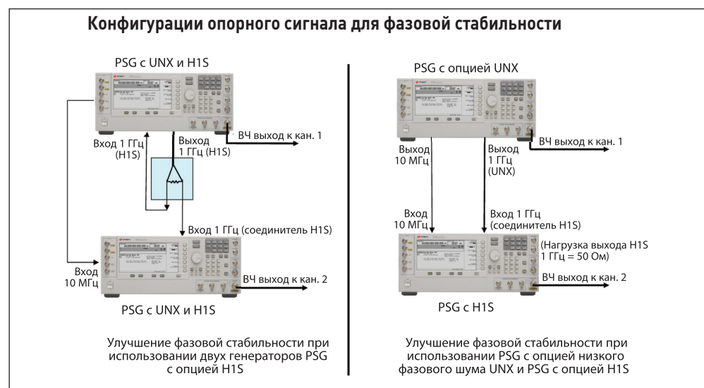
Рисунок 11. Опции H1S, H1G и UNX генератора PSG позволяют улучшить фазовую стабильность между приборами с помощью синхронизации опорным сигналом с частотой 1 ГГц.
