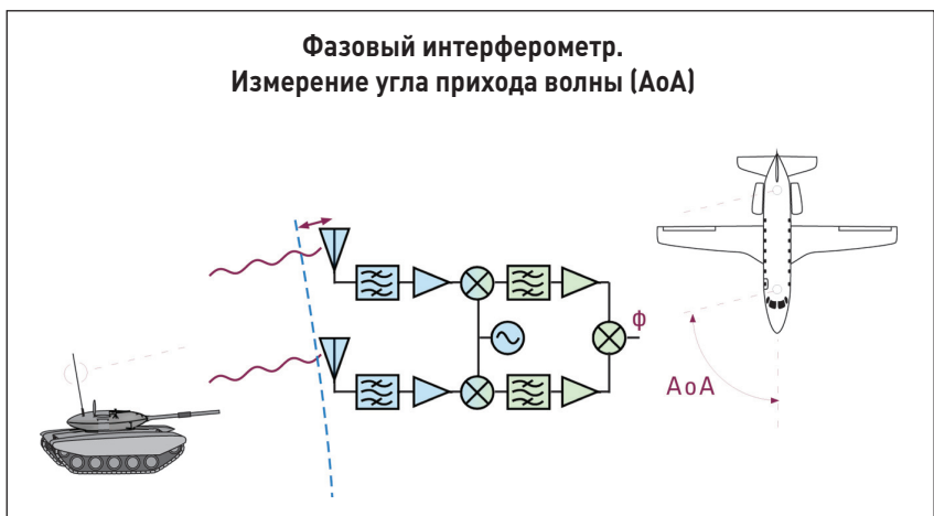
Рисунок 1е. Система определения направления может определять угол прихода волны передаваемого сигнала путём измерения фазовой задержки между двумя пространственно-разнесёнными приёмниками.
