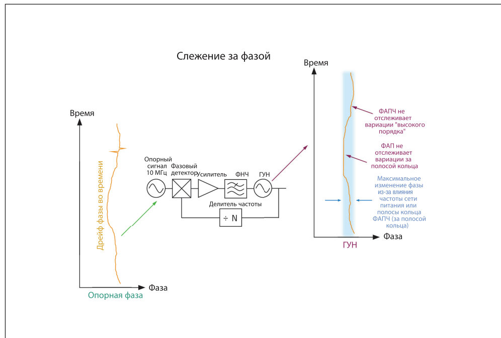
Рисунок 6. Системы ФАПЧ обычно хорошо, но не совершенно отслеживают фазу источника сигнала, но не способны отслеживать вариации фазы более высокого порядка.
