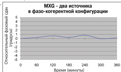
Рисунок 7. Результаты измерения дрейфа фазы двух генераторов MXG, синхронизированных опорным сигналом 10 МГц, в сравнении с двумя когерентно синхронизированными генераторами MXG (использующими общий гетеродин).
