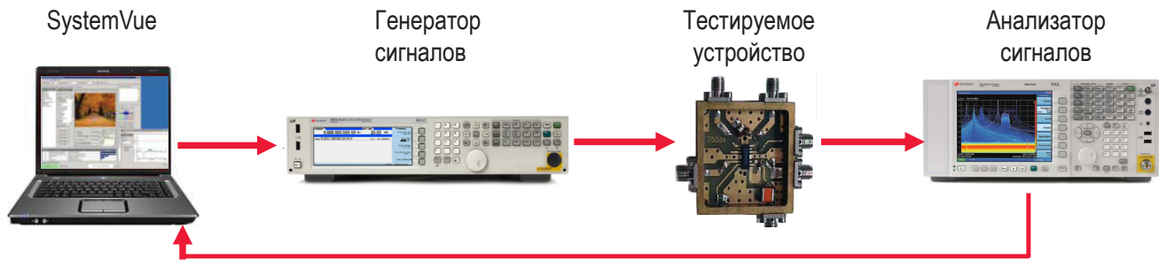
Рисунок 13 – Пример комбинации программных средств и измерительных приборов, которая может быть использована для создания и генерации испытательных сигналов РЛС
