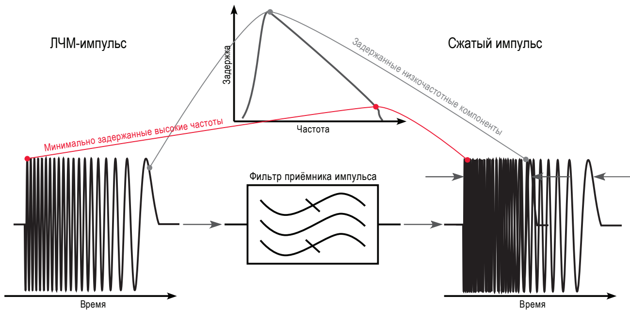
Рисунок 2 – Сжатие ЛЧМ импульса
