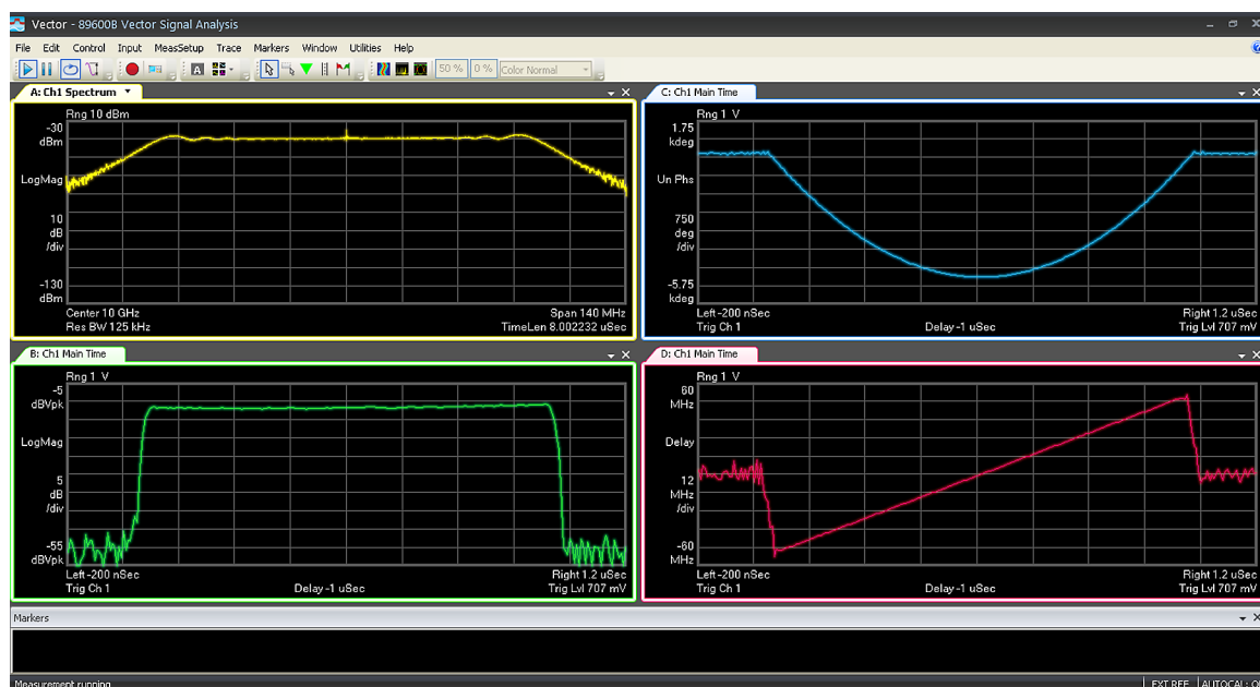
Рисунок 17 – Просмотр ЛЧМ-импульса с помощью программного обеспечения 89600 VSA
