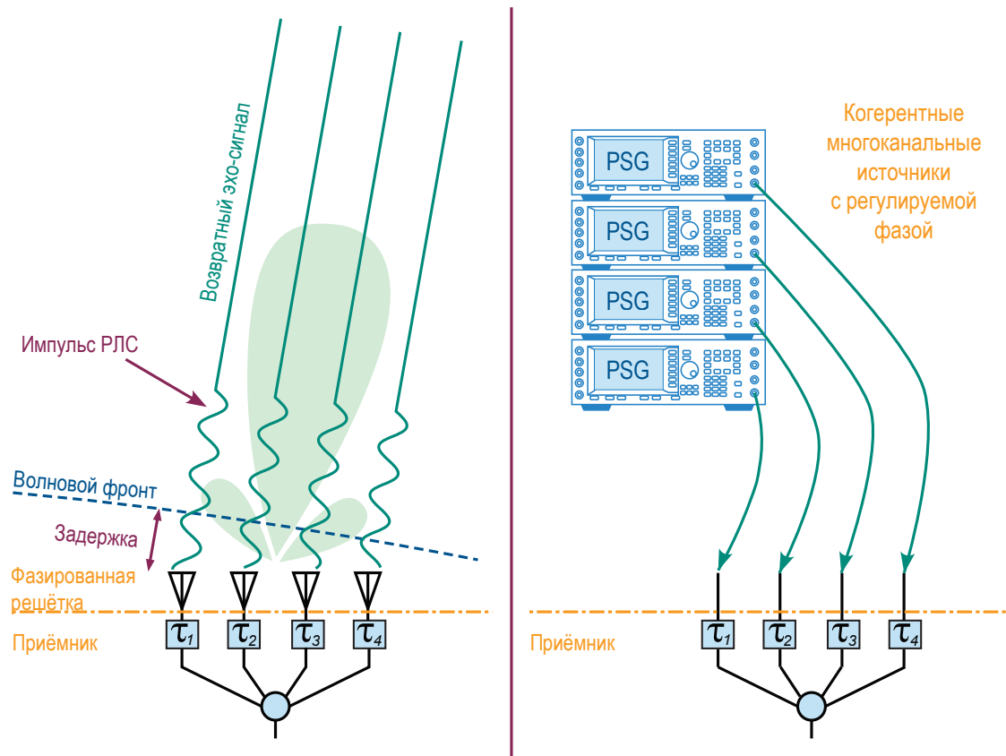
Рисунок 11 – Создание искусственного испытательного полигона для РЛС с фазированной антенной решёткой
