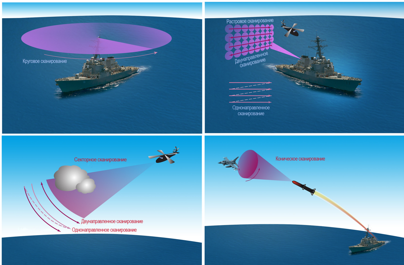
Рисунок 8 - Диаграммы сканирования антенн
