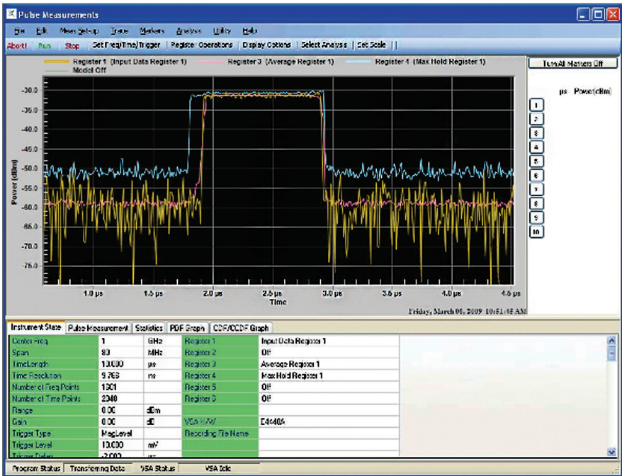
Рисунок 18 – Программное обеспечение для измерения параметров импульсов N9051A
