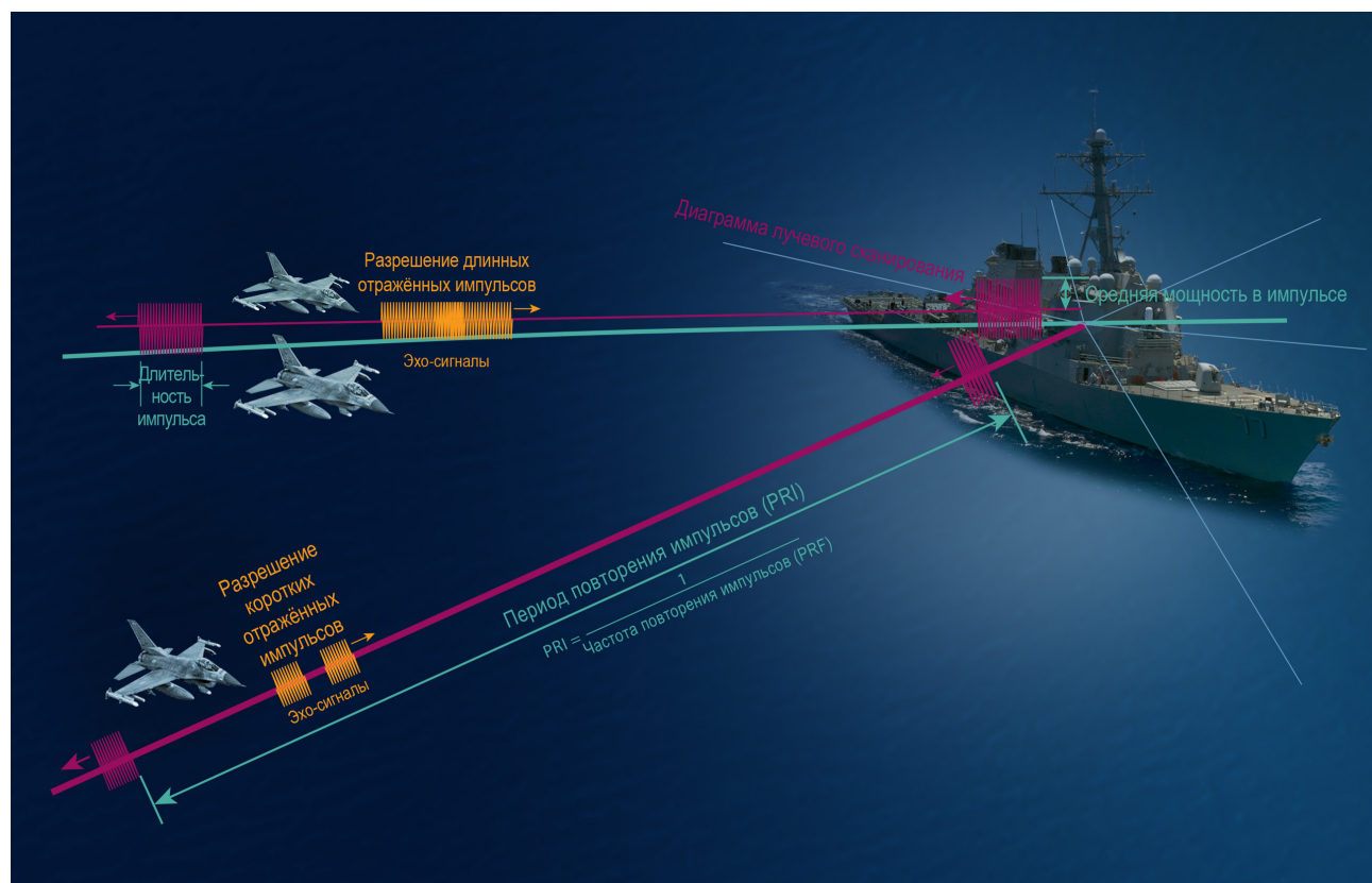
Рисунок 1 – Термины и соотношения, относящиеся к импульсу РЛС
