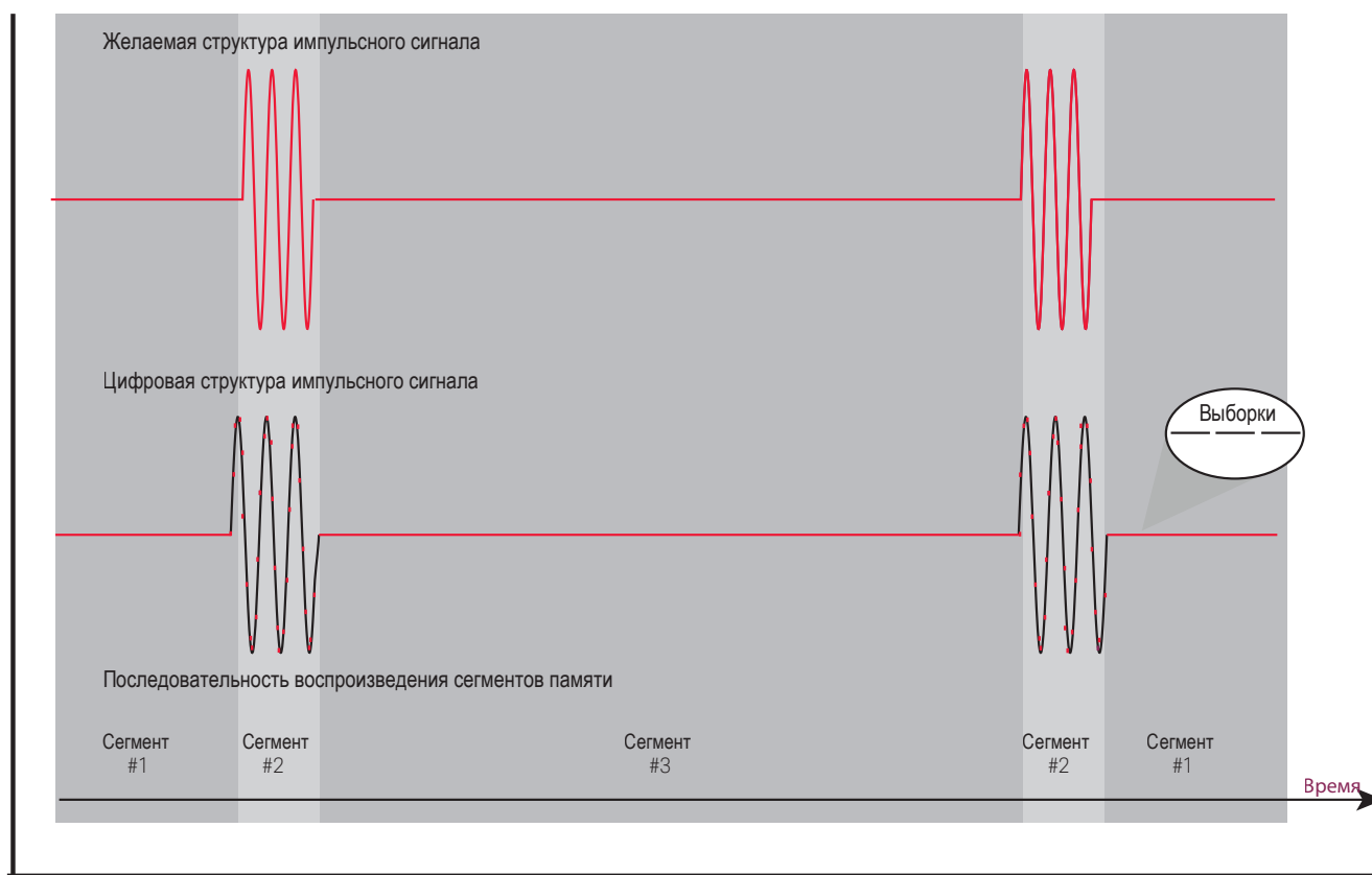
Рисунок 6 - Сегментирование сигнала, формирование последовательностей и сценариев
