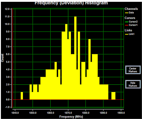
Рисунок 19 – Углублённый анализ импульсов с использованием программного приложения для осциллографического анализа сигналов (OSA) W2650A включает возможность определения статистических характеристик с помощью гистограмм.
