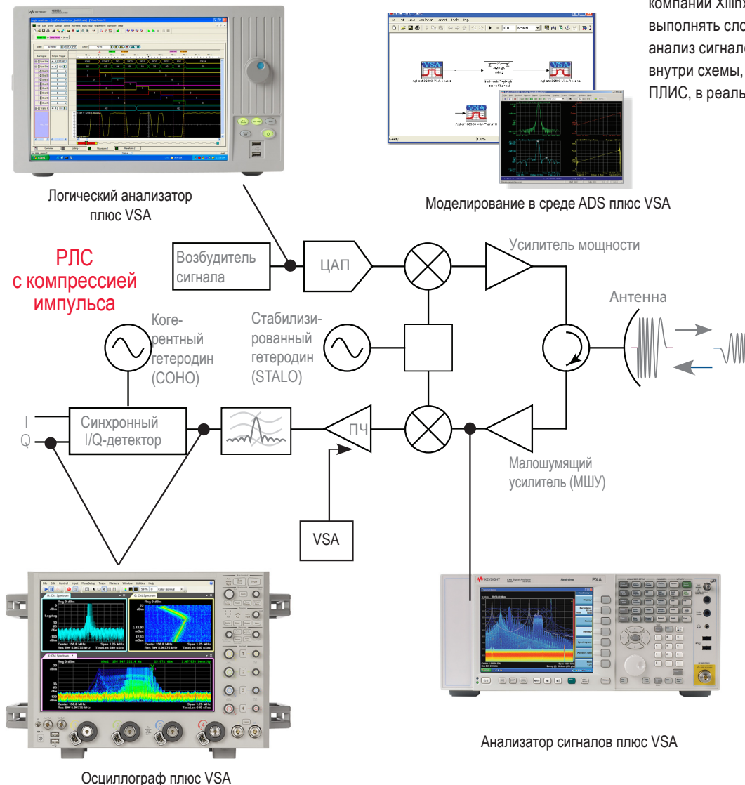
Рисунок 20 – Многоформатный анализ с помощью 89600 VSA
