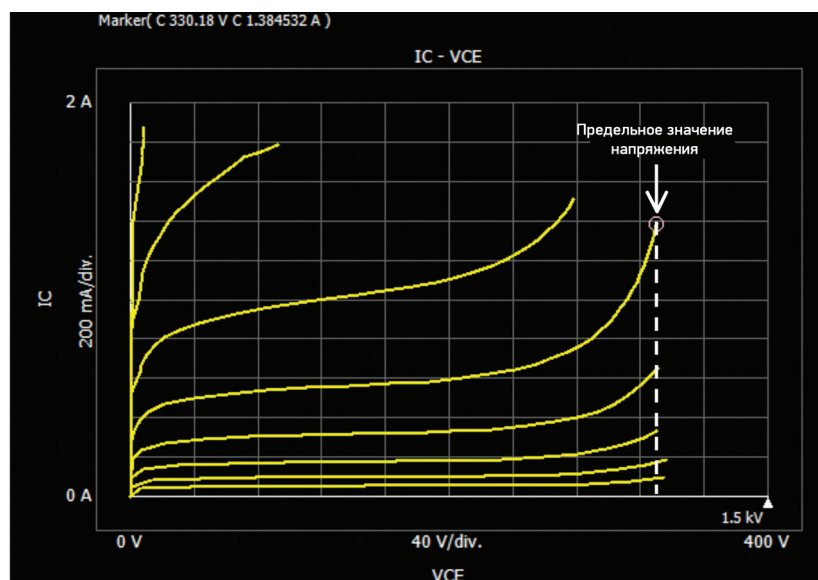
Рисунок 5. Характеристики БТИЗ вблизи пробоя (HVMSU).
