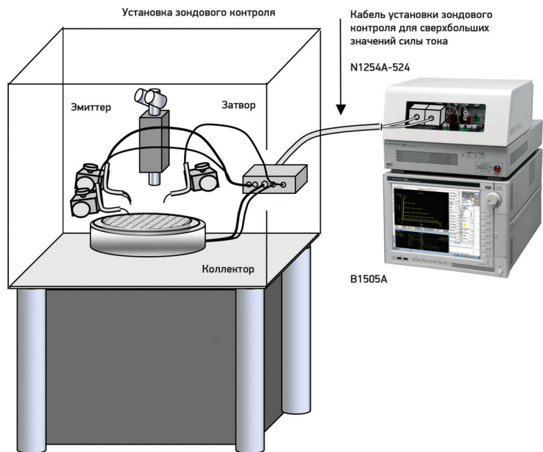
Рисунок 10. Подключение к установке зондового контроля с использованием кабеля установки зондового контроля для сверхбольших значений силы тока N1254A-524.
