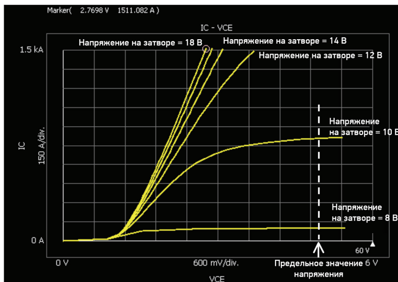
Рисунок 3. Характеристики БТИЗ в открытом состоянии (UHCU).
