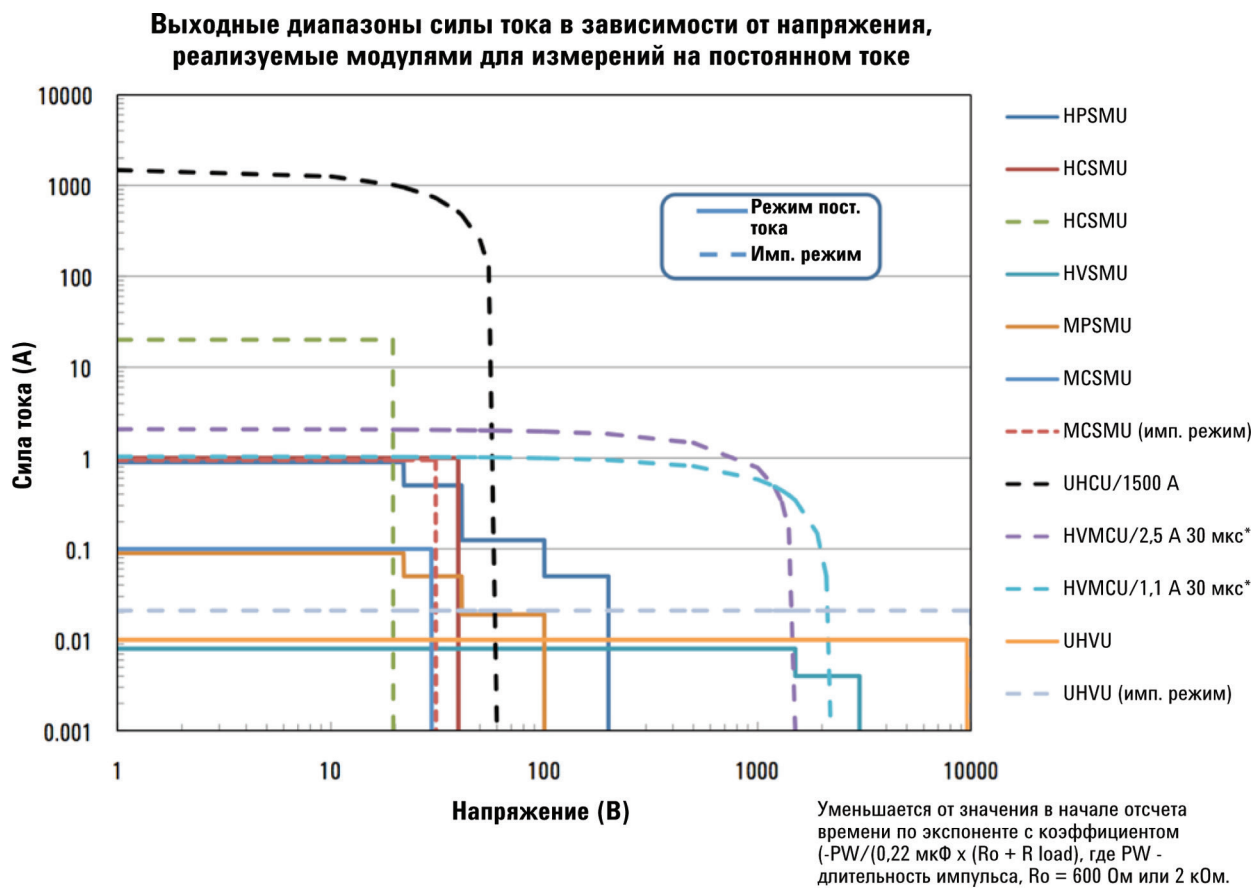
Рисунок 1. Выходные диапазоны силы тока анализатора B1505A.
