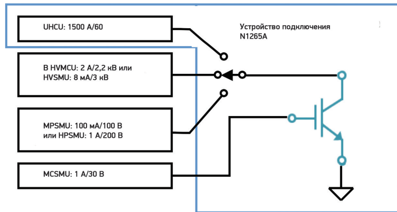
Рисунок 9. На тестируемое устройство (ТУ) можно подать до 1500 А и 3 кВ без какого-либо изменения кабельных соединений.
