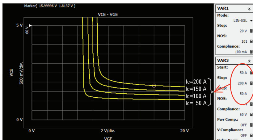
Рисунок 4. Характеристики зависимости напряжения коллектор-эмиттер от напряжения затвор-эмиттер ( V_{ce} - V_{ge} ) БТИЗ в открытом состоянии (UHCU).
