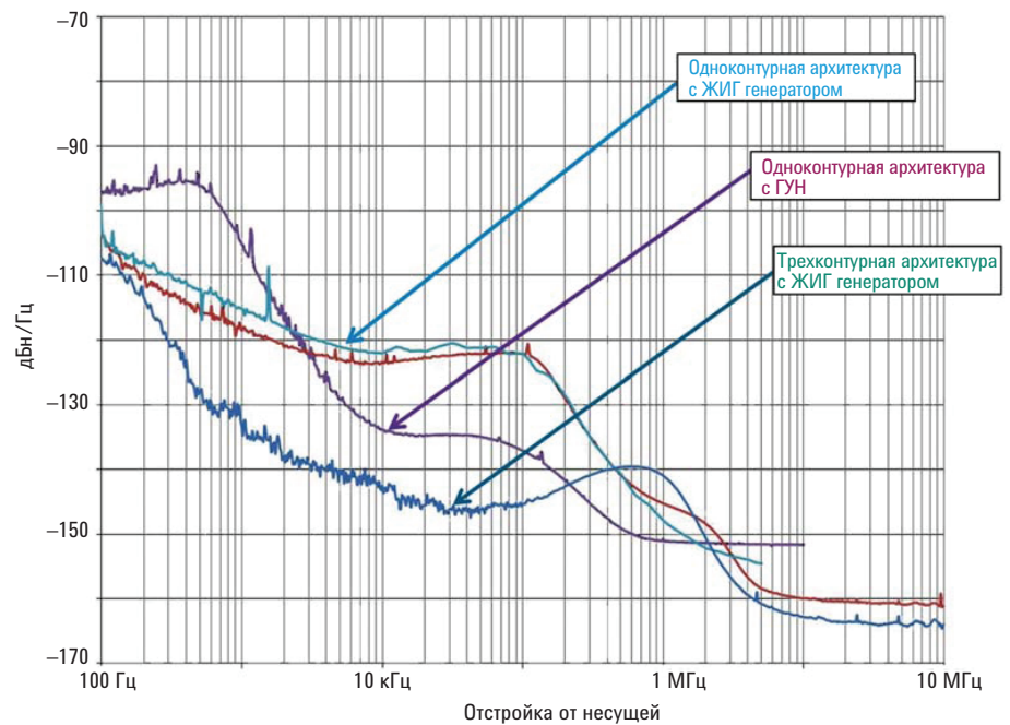
Рис. 5. Комбинация архитектуры и типа гетеродина влияет на общее значение фазового шума, а также на зависимость фазового шума от отстройки и частоты.
