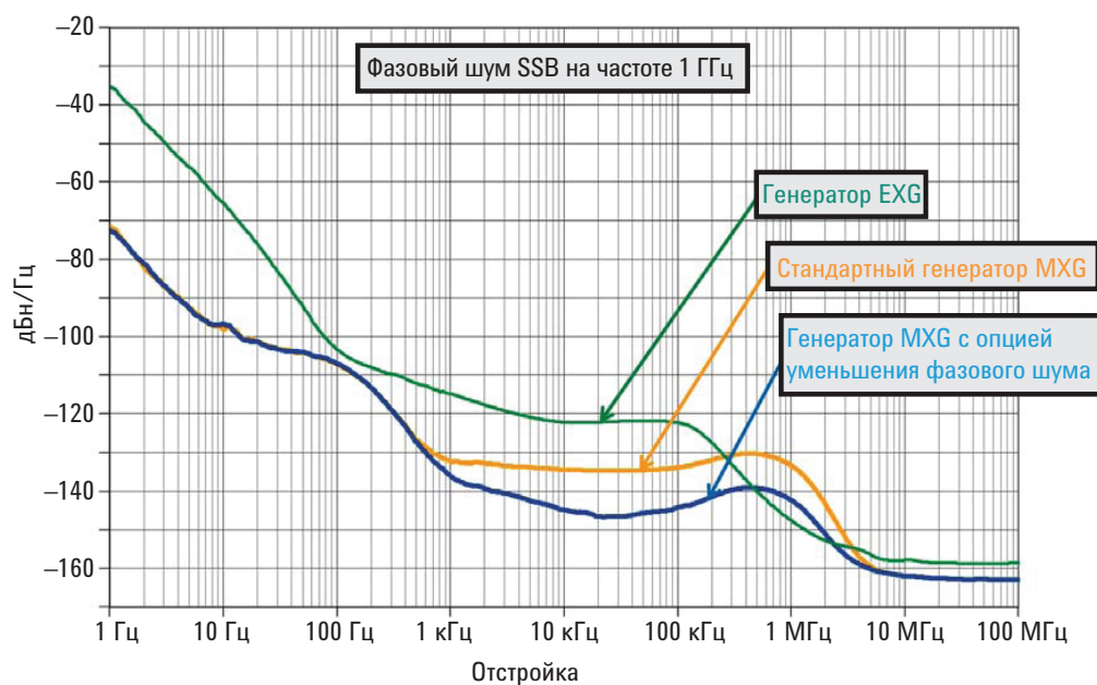
Рис. 4. Одноконтурный генератор EXG подходит для многих приложений, а многоконтурный генератор MXG можно эффективно использовать для более точных измерений.
