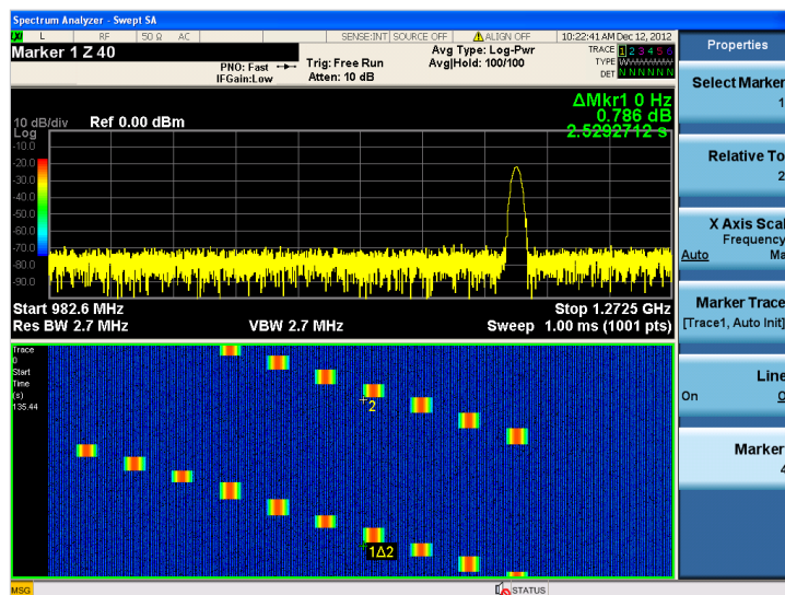
Рисунок 5. Отображение спектрограммы на экране приёмника MXE.
