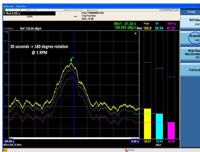
Рисунок 4. Отображение измерения приёмника MXE в виде ленточной диаграммы.
