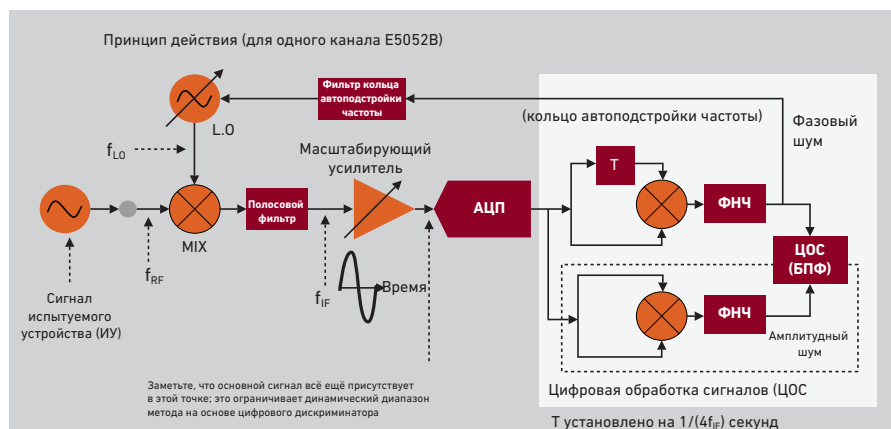
Рисунок 6 - Цифровые технологии позволяют имитировать поведение аналоговой линии задержки и проводить точные измерения фазового шума.
