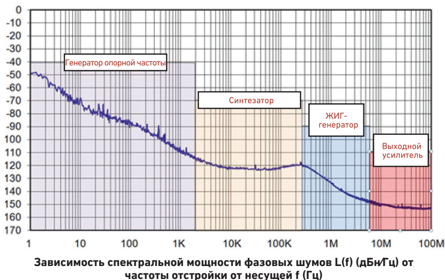
Рисунок 2 - Составляющие характеристик фазового шума генератора сигналов могут быть отслежены и сопоставлены с основными блоками его внутренней архитектуры.
