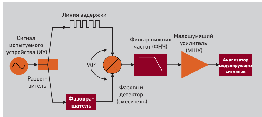
Рисунок 5 - Разветвление сигнала ИУ и манипулирование им с помощью линии задержки и фазовращателя исключает необходимость в опорном источнике..
