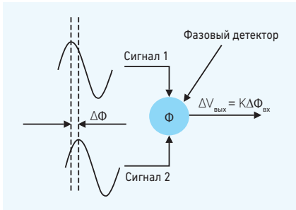
Рис. 3. Функциональная схема фазового детектора, используемая во многих приборах.
