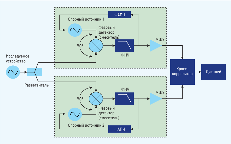
Рис. 4. В анализаторе E5052B метод двухканальной кросс-корреляции реализуется с помощью двух фазовых детекторов.
