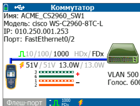
Соединение 100 Мбит/с с PoE на порте 2 по медной линии
