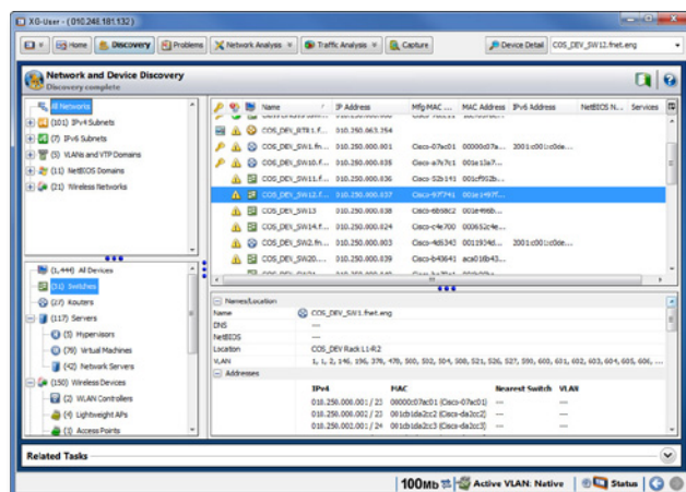
Обнаружение устройств и сети
