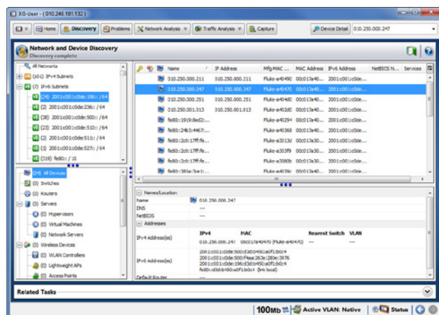
Сети IPv6, приложения и устройства
