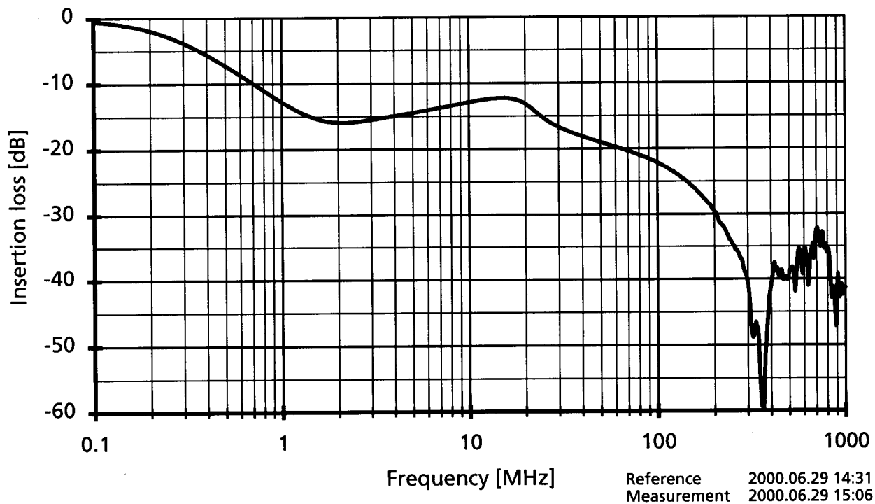
Typical insertion loss in a 50 Ω system Typische Dämpfung in einem 50 Ω System
