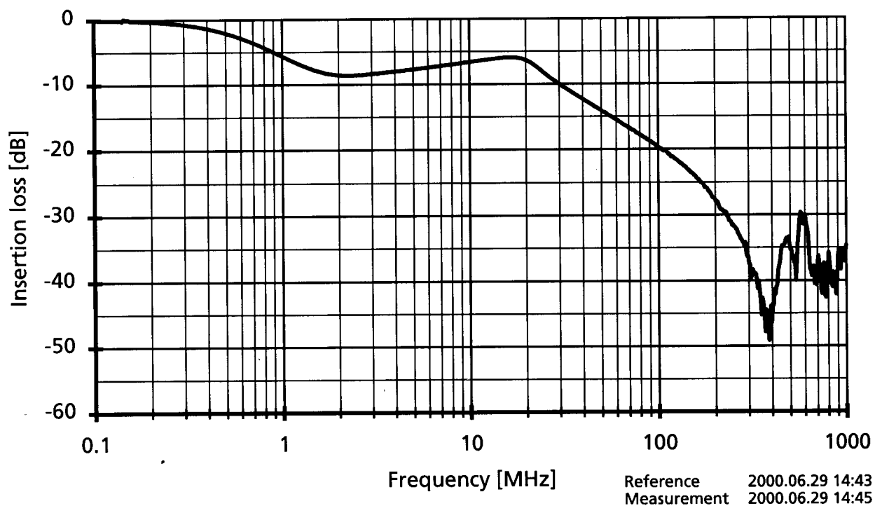
Typical insertion loss in a 150 Ω system Typische Dämpfung in einem 150 Ω System
